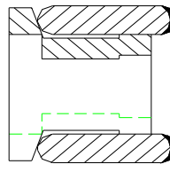
TPR - OD CHROME RAILS H' TYPE EXPANDER CODE : 307
